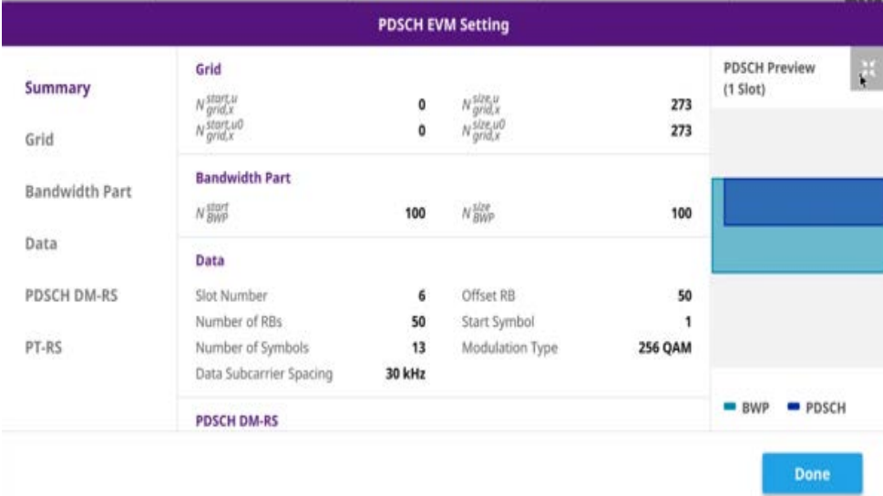
Figure 136 5G NR PDSCH EVM setting summary
